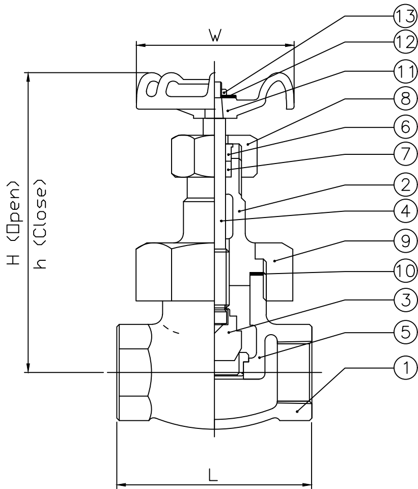
詳細尺寸 Dimension 單位 Unit: 公釐 mm
