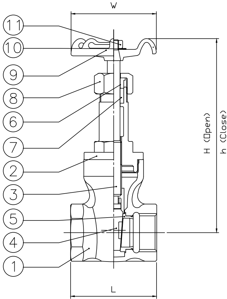
詳細尺寸 Dimension 單位 Unit: 公釐 mm
