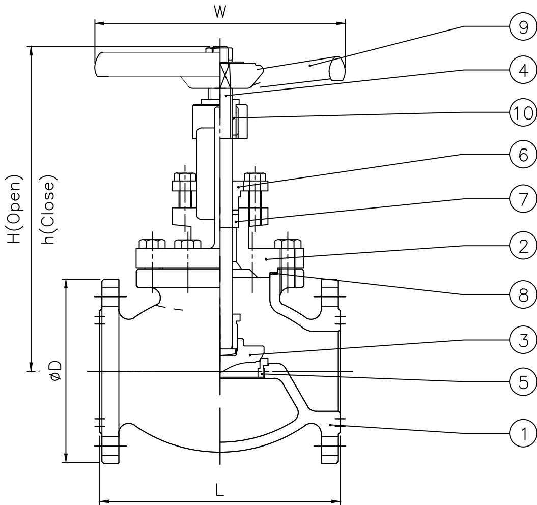
詳細尺寸 Dimension 單位 Unit:公釐 mm
