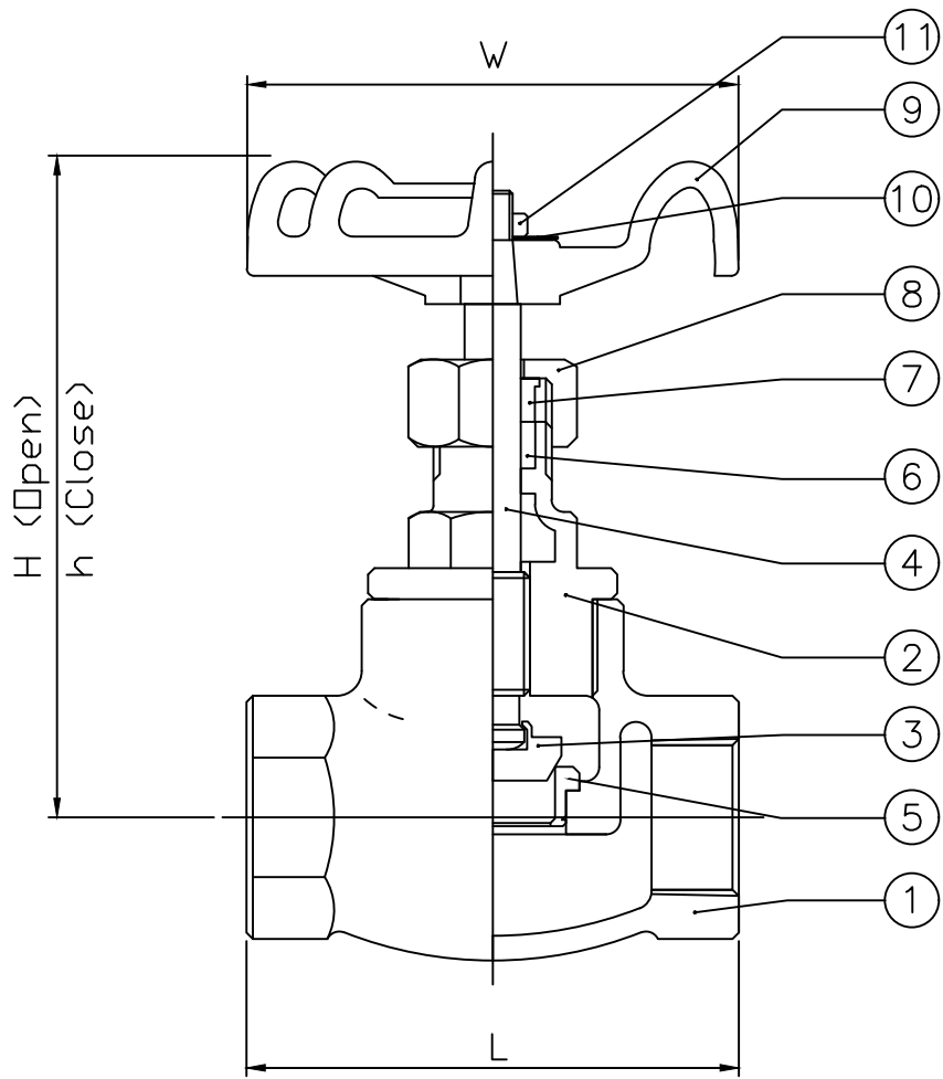
詳細尺寸 Dimension 單位 Unit: 公釐 mm
