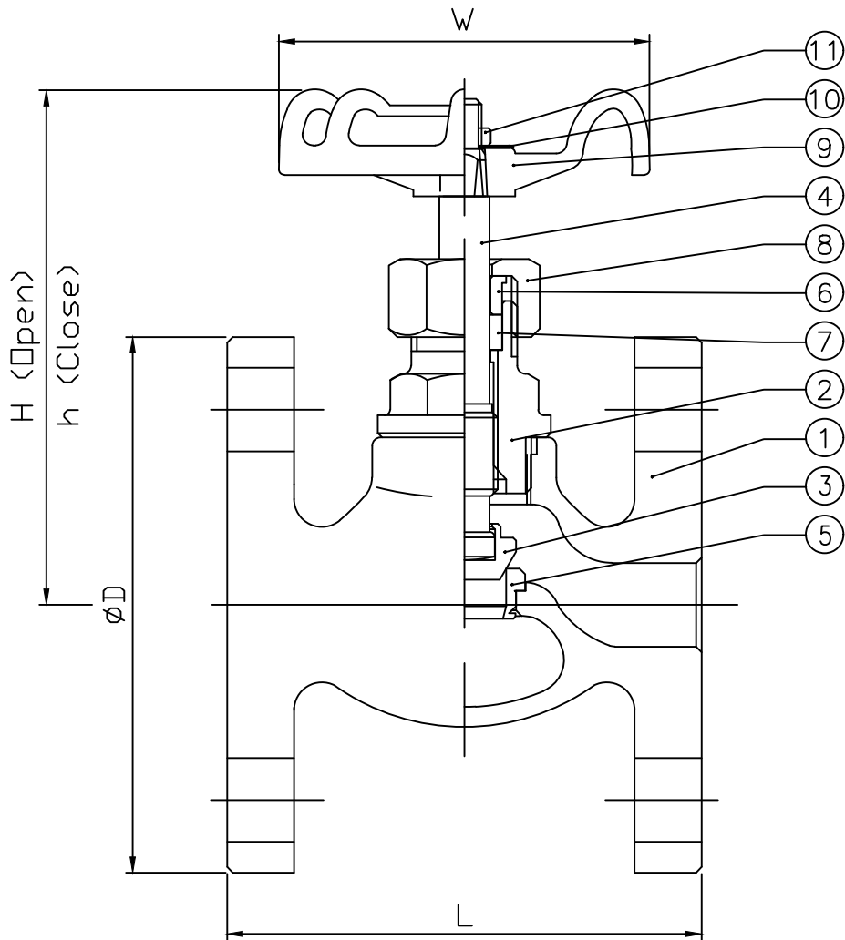
詳細尺寸 Dimension 單位 Unit: 公釐 mm
